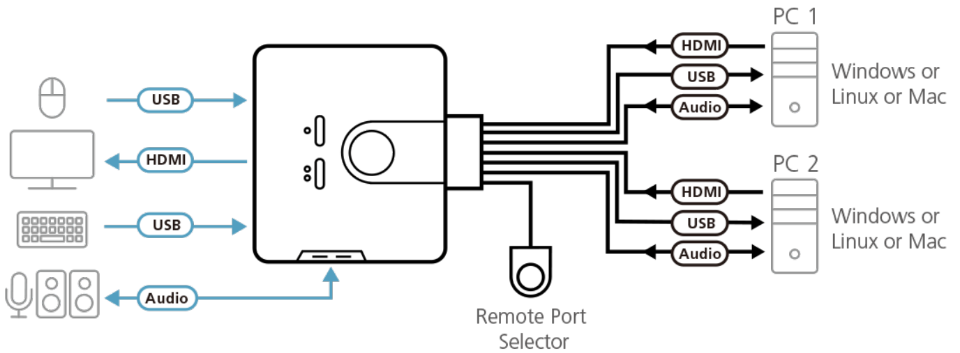
構成図
