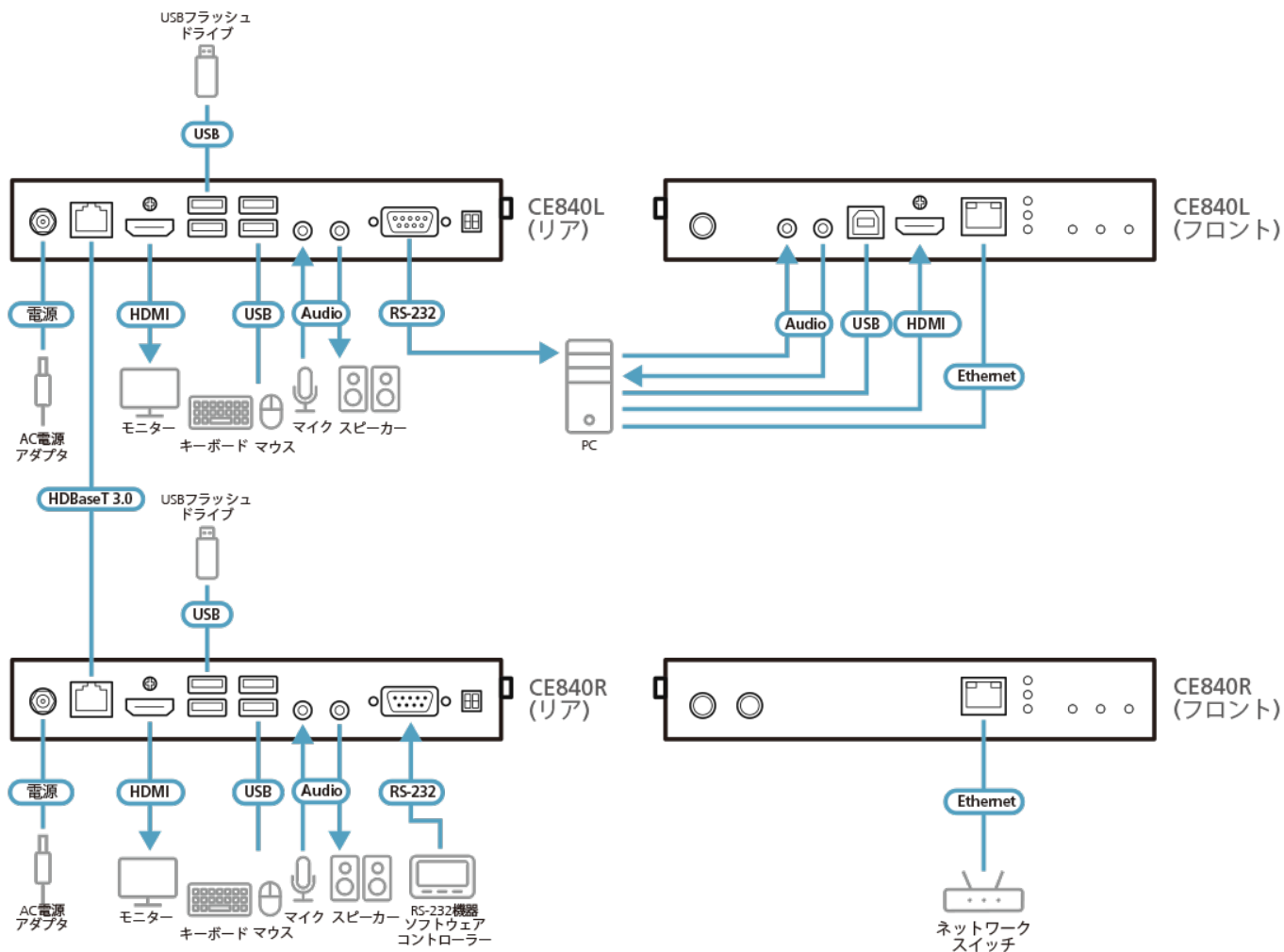
構成図
