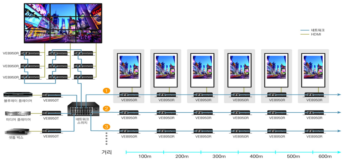
데이터체인을 사용하여 비디오 월을 구성하거나 A/V시스템을 수백 미터 확장합니다.
