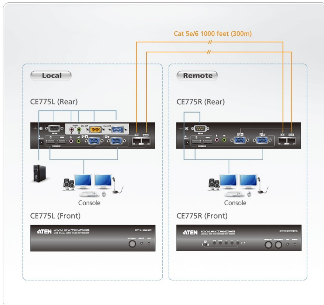
連線圖
